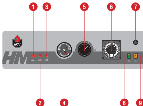
Panel de mandos de la HeatMaster® 30 N y 60 N
