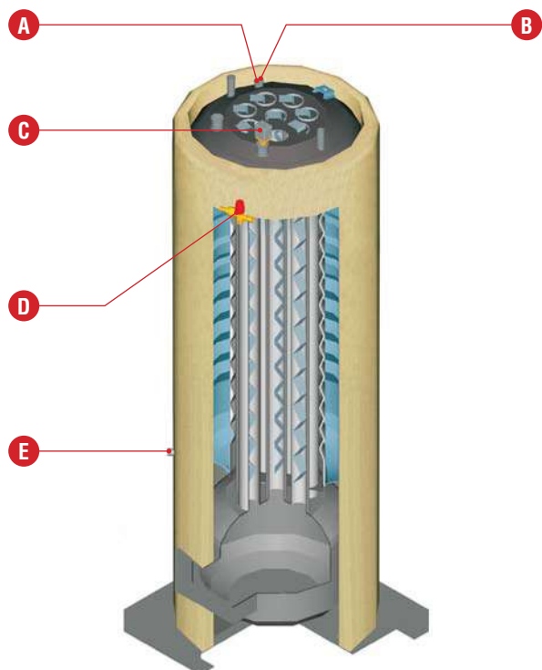
Características de seguridad de la HeatMaster® 30 N y 60 N
